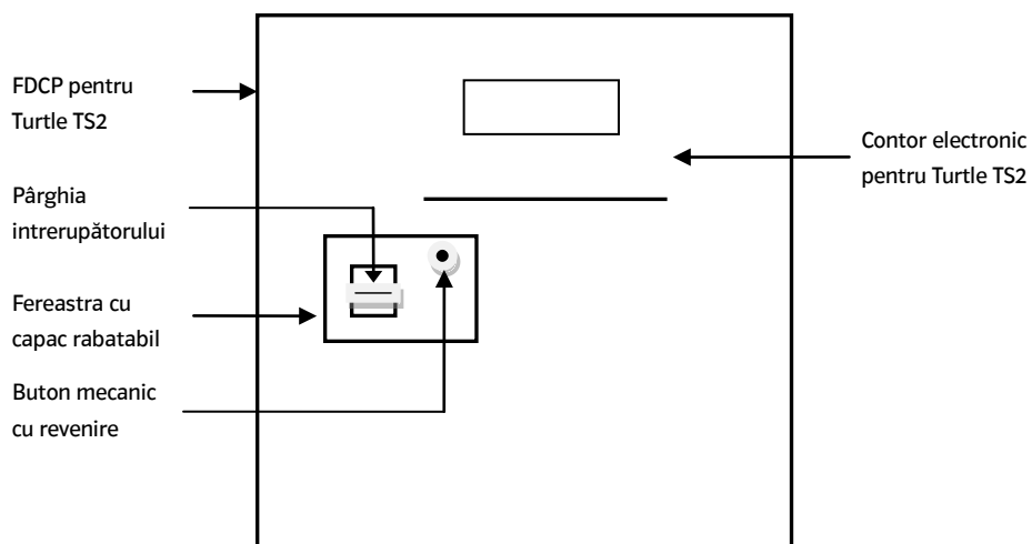
Fig.3 Desen cu decupaj din FDCP pentru contoare electronice monofazate integrabile în sistemul Turtle TS2. Poziționarea ferestrei cu capac rabatabil.
