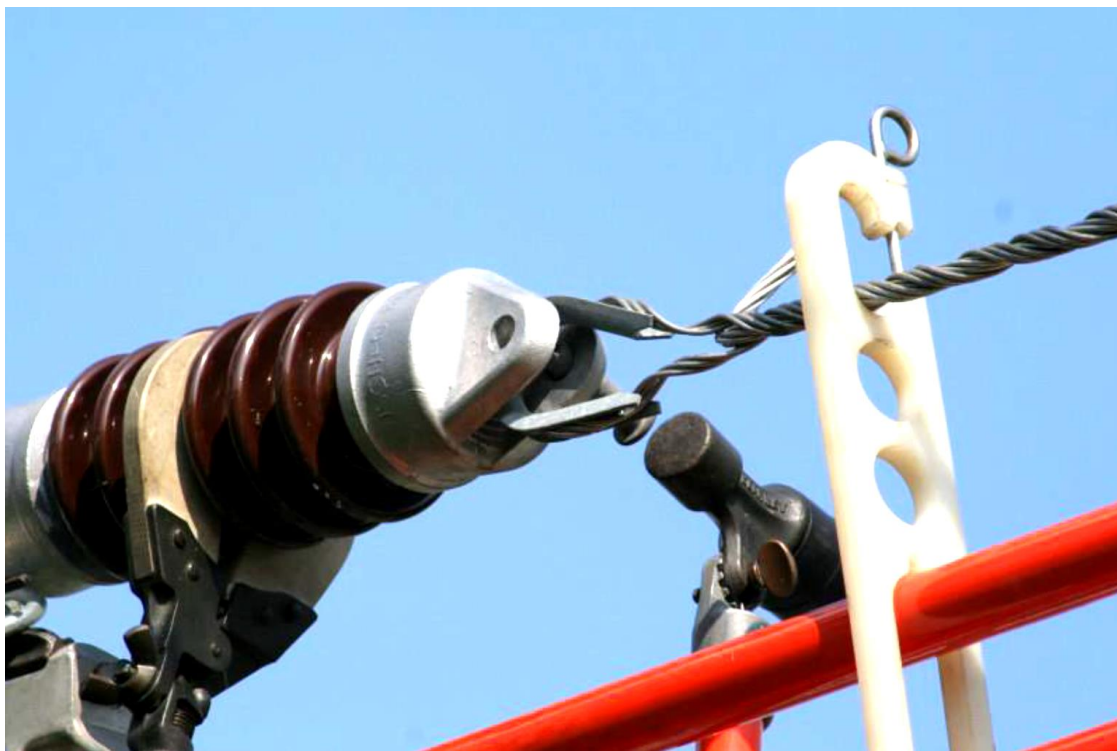
Exemplu de utilizare ciocanului pentru montarea unui bolt la un izolator de întindere
