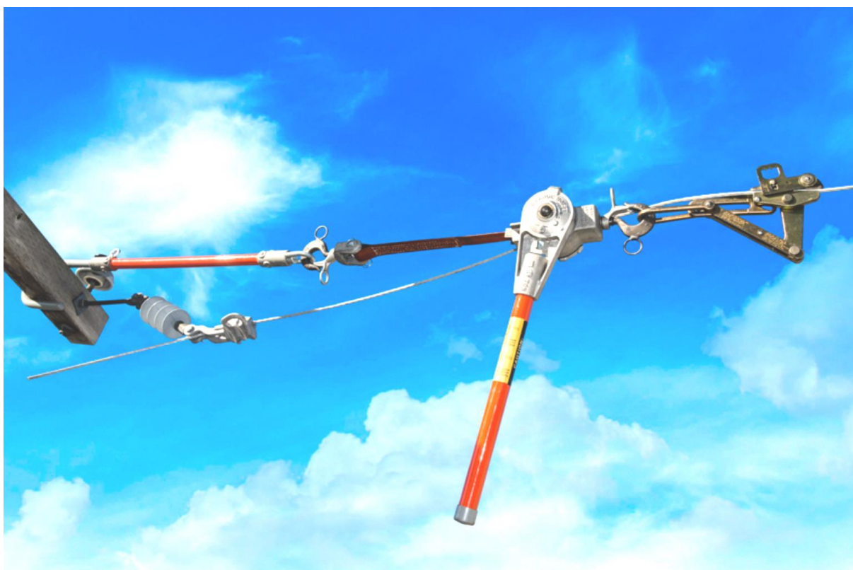
Exemplu de utilizare a unui palan cu chingă pentru detensionarea unui izolator de întindere.
