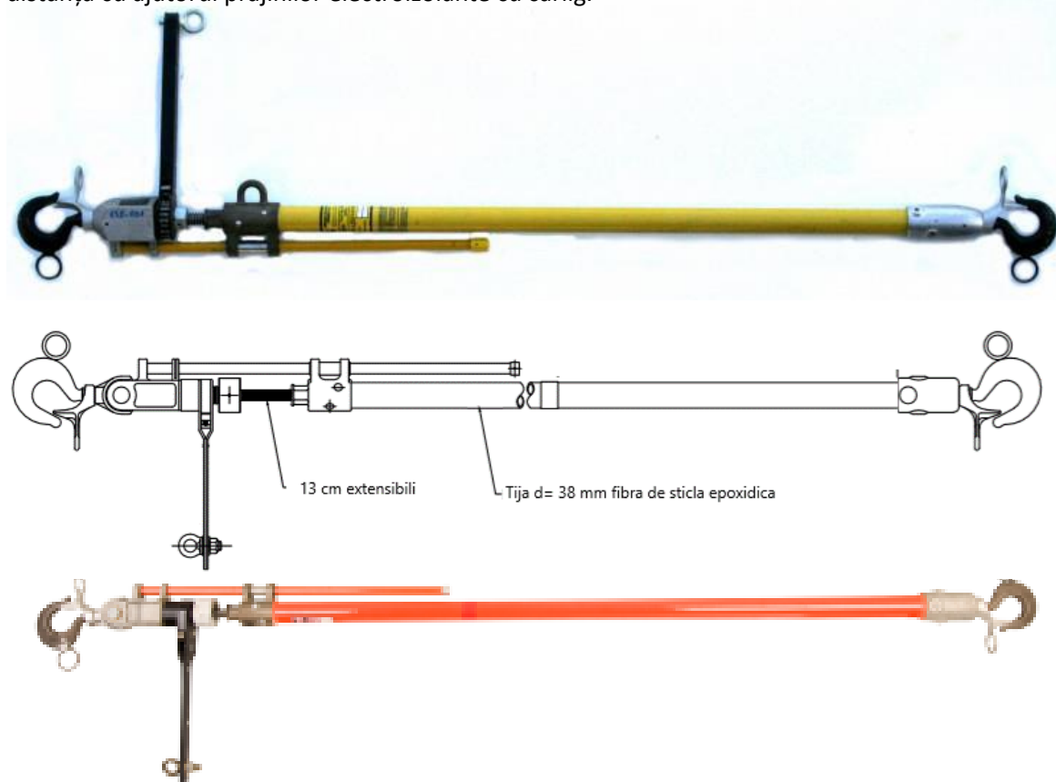
Exemple de tiranți simpli de detensionare
