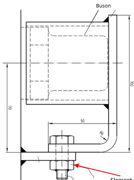
Fig. 3 Protecție mecanică a bușonului de golire
