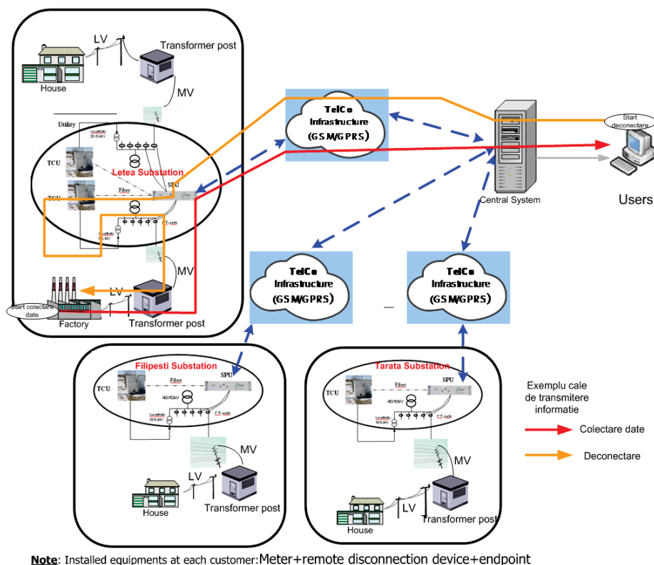
Figura 1 Schema de principiu a sistemului TURTLE TS2
