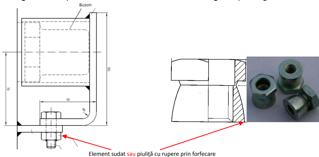
Fig. 3 Protecție mecanică a bușonului de golire
