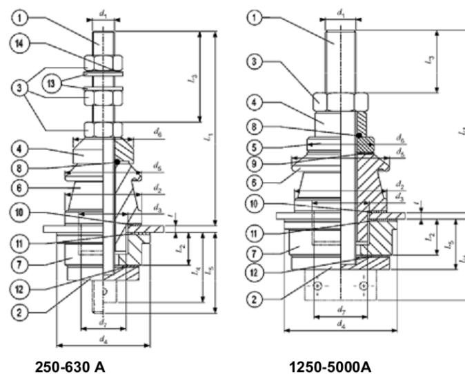
Fig. 4 Izolatoare JT
